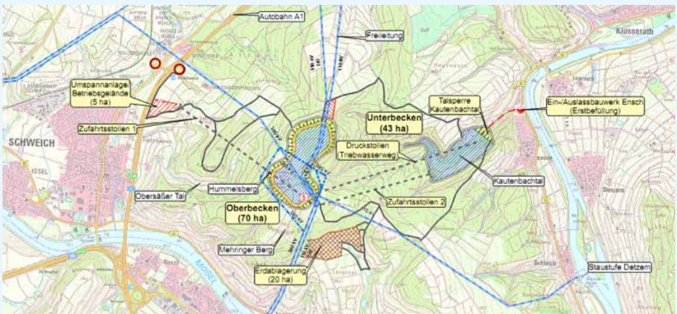
Abb. 24: Geplante Lage des Pumpspeicherwerks Rio – Quelle: Raumordnungsverfahren
